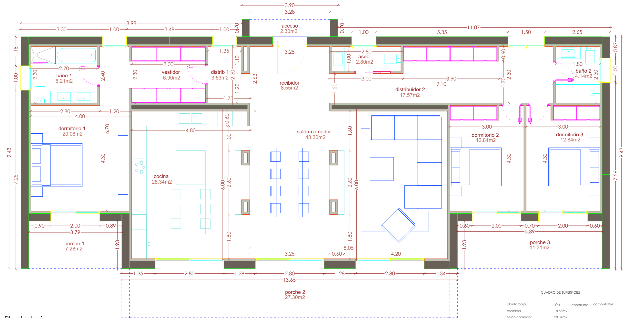
Planta baja
